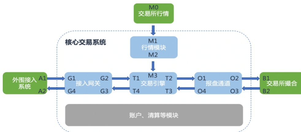
图1 核心交易系统参考架构图
